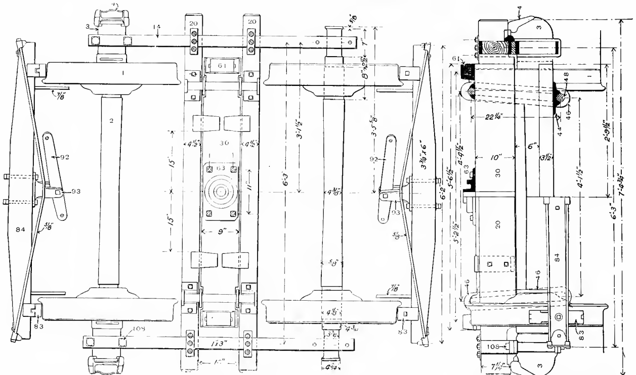
Fig. 4751. Plan.
